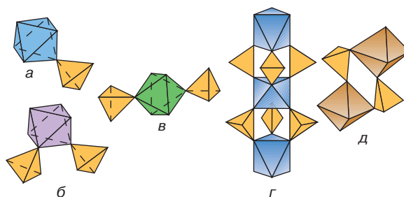
Рис. 5. Изолированные структурные единицы в структурах сульфатных минералов: а – димеры в минасрагрите \text{VO}_2\text{SO}_4 \cdot 5\text{H}_2\text{O} ; б – тримеры в ремерите \text{Fe}^{2+}\text{Fe}^{3+}(\text{SO}_4)_4 \cdot 14\text{H}_2\text{O} ; в – тримеры в бледите \text{Na}_2\text{Mg}(\text{SO}_4)_2 \cdot 4\text{H}_2\text{O} ; г – линейный комплекс в кокимбите \text{Fe}_2(\text{SO}_4)_3 \cdot 9\text{H}_2\text{O} ; д – кольцо из двух \text{SO}_4 -тетраэдров и двух Mg-октаэдров в структуре старкеита \text{MgSO}_4 \cdot 4\text{H}_2\text{O}
